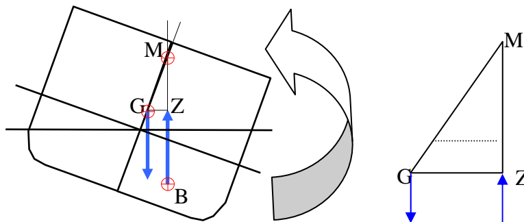
Slagzij maken
